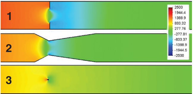
三种压损比较：（1）孔板；（2）文丘利管；（3）西斯特德尔塔巴流量计探头
